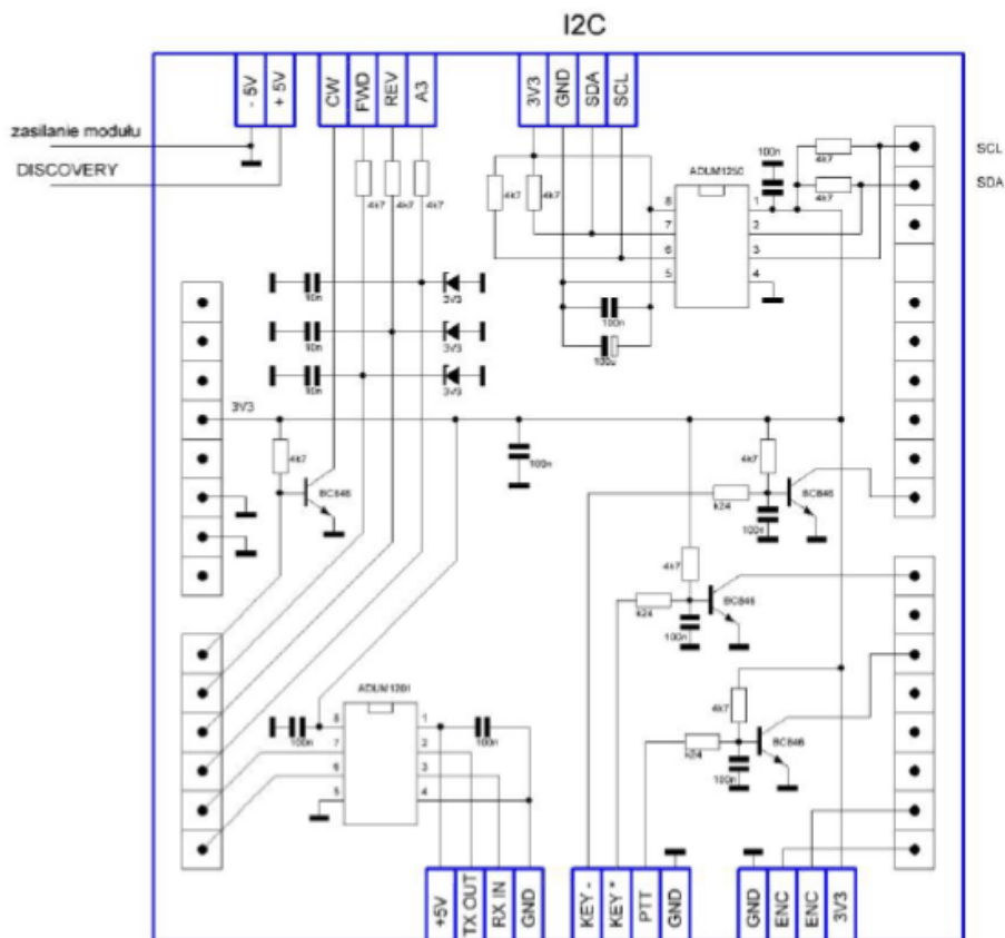
Schemat adaptera V6. rys. sp5bmp 04/2017
